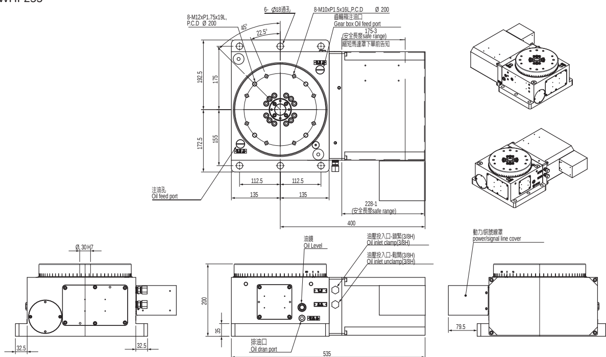
SWHI-255
